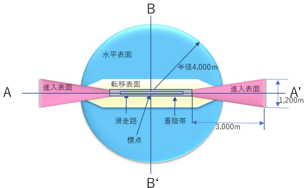
平面概略図
